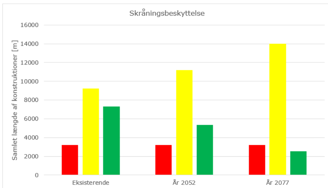
Figur 5.1 Tilstandsvurdering af skråningsbeskyttelser i dag (eksisterende), år 2052 og 2077, ved en strandfodring med ral til kote +1,2 m og ovenpå rallen sand til kote +1,5 m. Strandfodringen forudsættes vedligeholdt og udbygget for at fastholde vanddybden foran konstruktionerne. Grøn: Vurderet at opfylde forudsætningerne. Gul: Vurderet at opfylde forudsætningerne efter forhøjelse. Rød: Vurderet at skulle genopbygges med større dæksten.
