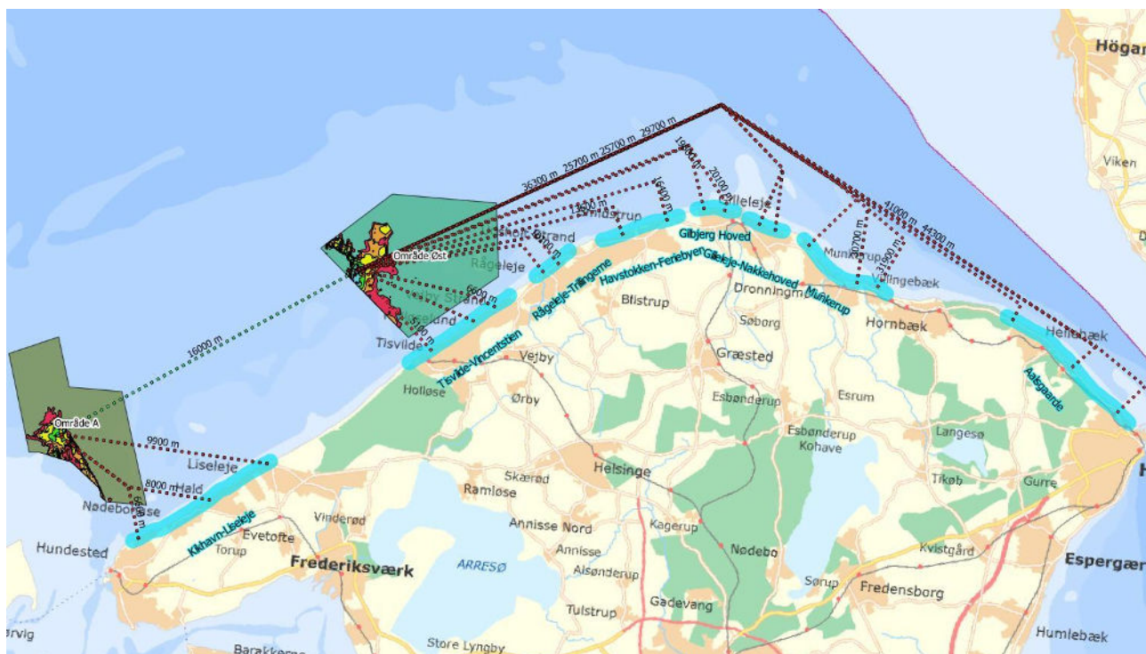
Figur 6.13 Sandindvindingsområders placering med sejlaflstande (stiplede linjer med afstand i m) til de analyserede kystprofiler i fodringsområderne (turkis markering).
