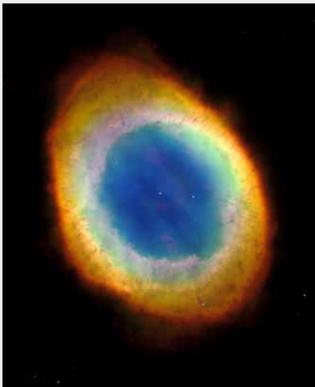
Den planetariske tåge Messier 57, optaget med Hubble rumteleskopet 16. oktober 1998. Vi kan ikke se farverne i en kikkert, fordi de celler i øjnene, som kan se svagt lys, ikke kan se farver. Foto: The Hubble Heritage Team (AURA/STScI/NASA/ESA).
